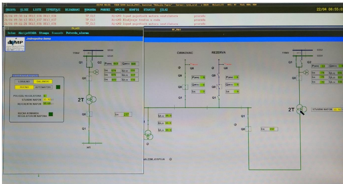
SLIKA 3 - DINAMIČKA SLIKA KOMPLETNOG 35 KV POSTROJENJA
